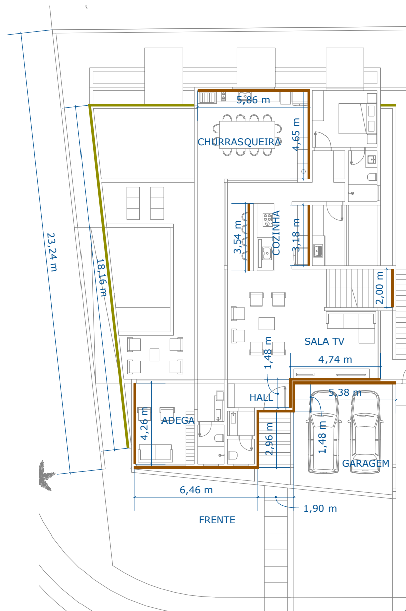
PLANTA TÉRREO Esc. 1:200
